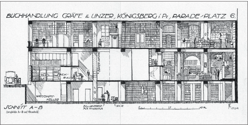
Schnitt, 1924.
