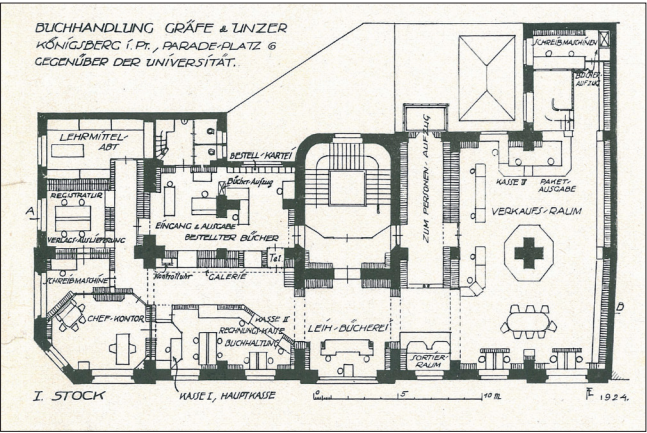
Grundriss 1. OG, 1924.
