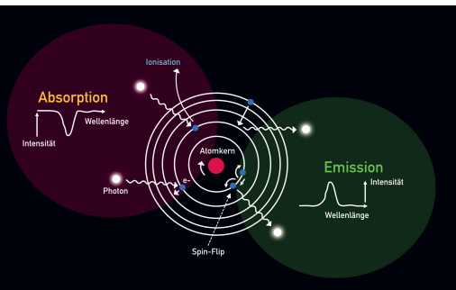
Schematische Darstellung der Entstehung von Spektrallinien durch die Absorption und Emission von Photonen in einem Atom.
